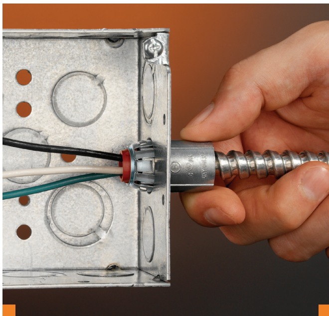
METAL CLAD CABLE
