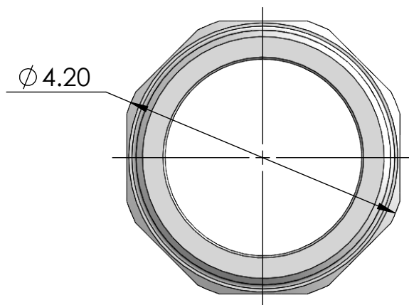
NUT
