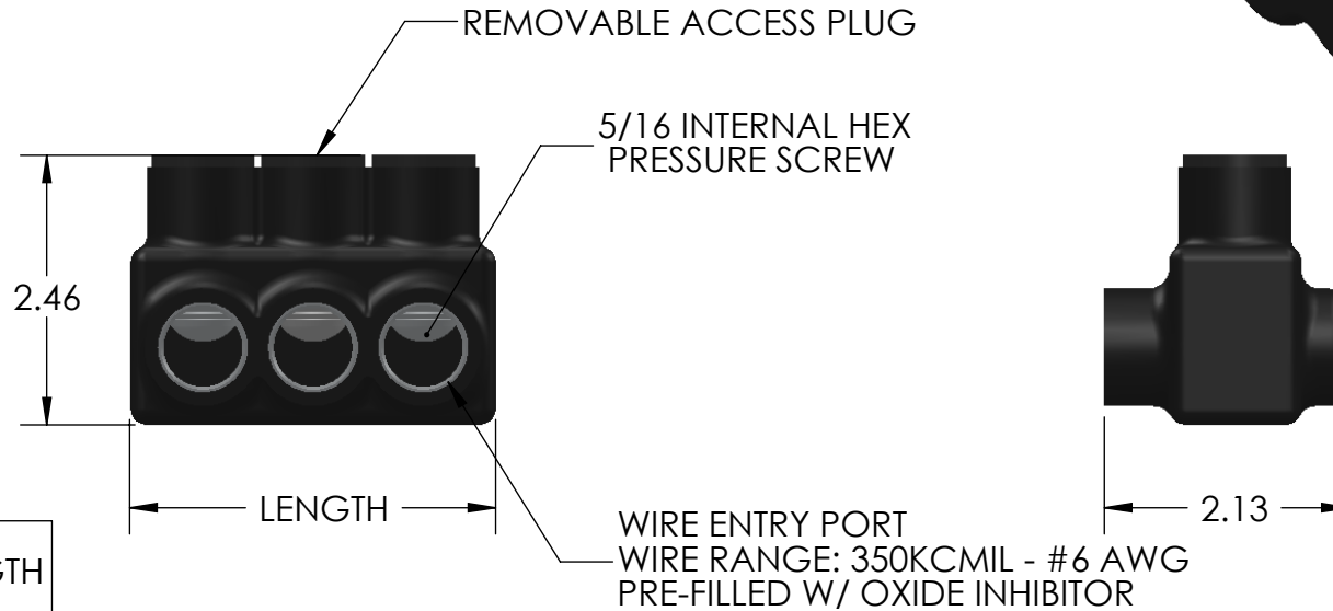
IPL350-3 SHOWN
