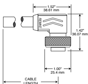
90° PLUG
