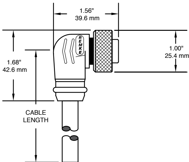
90° PLUG
