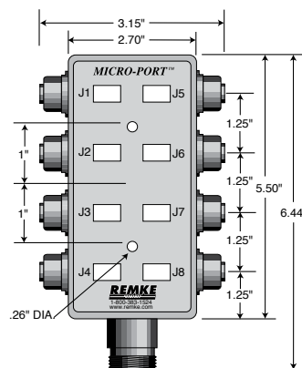
8 OUTLET
