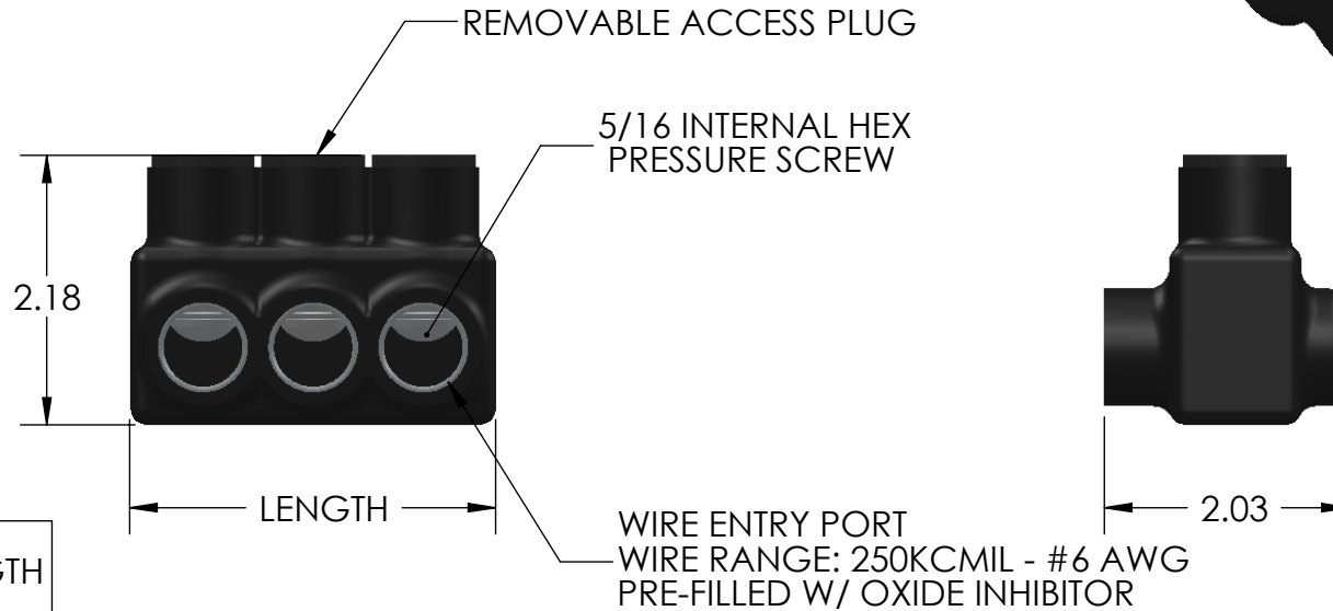
IPL250-3 SHOWN
