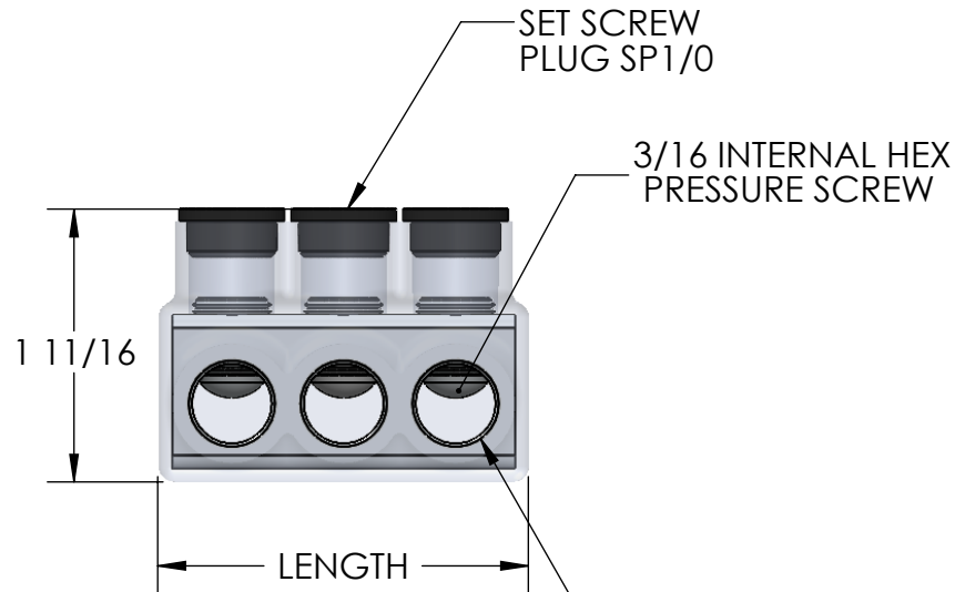
IPL1/0-3C SHOWN
